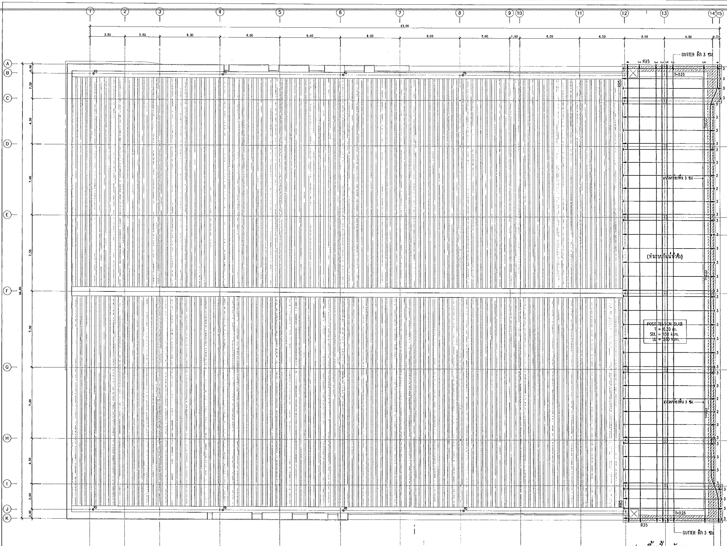
แปลนพื้นที่หลังคา SCALE 1:1,100 (TENDON LAYOUT)
