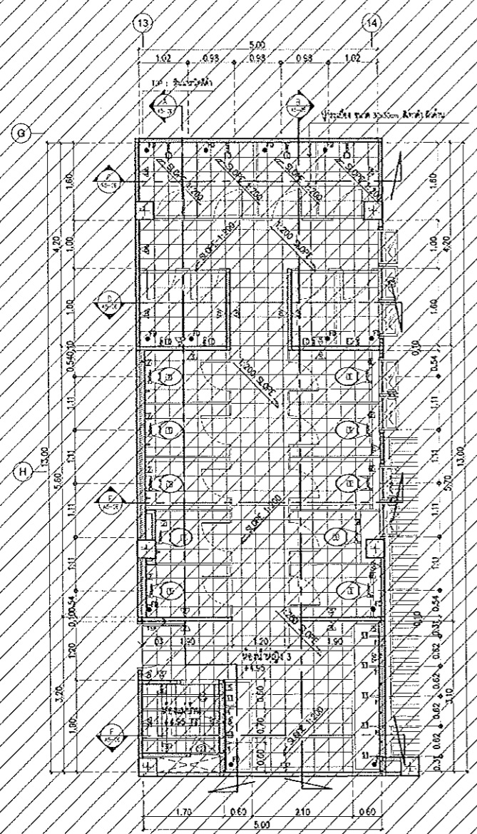
A5-06 แปลนขยายห้องน้ำหญิง 3 Scale 1:50
