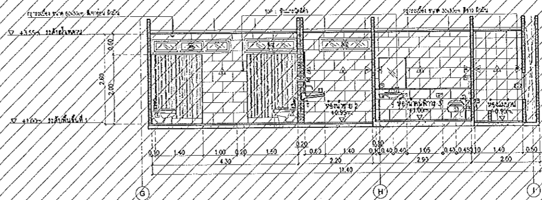
AS-04 AS-04 Scale 1:50 แบบขยายรูปตัด
