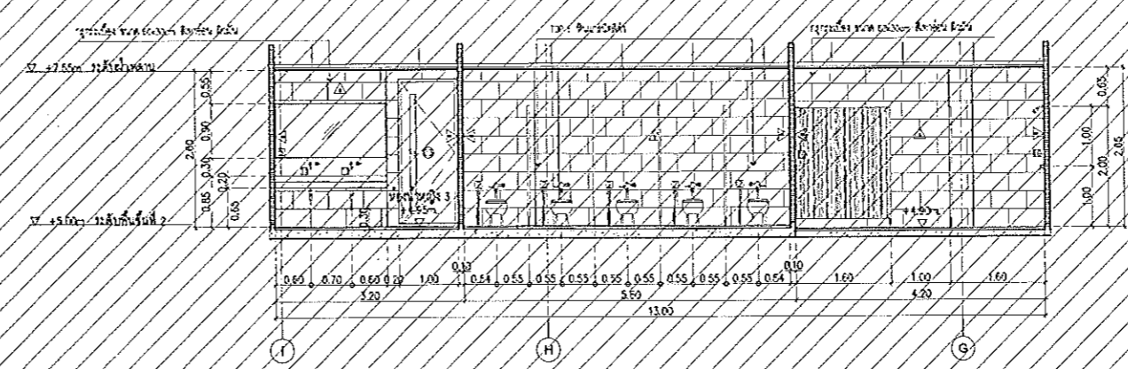
A5-06 แบบขยายรูปตัด Scale 1:50
