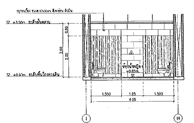
C แบบขยายรูปตัด A5-02 Scale 1 : 50
