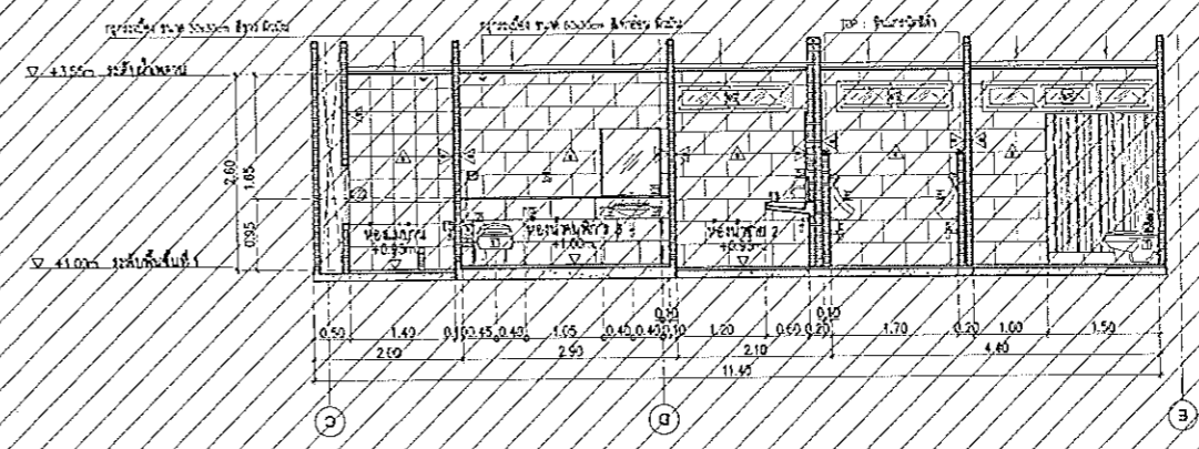
แบบขยายรูปตัด A-A Scale 1:50
