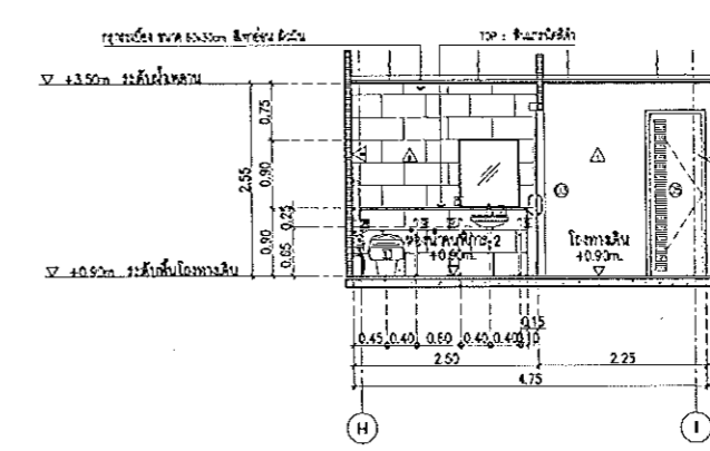
E แบบขยายรูปตัด A5-02 Scale 1 : 50
