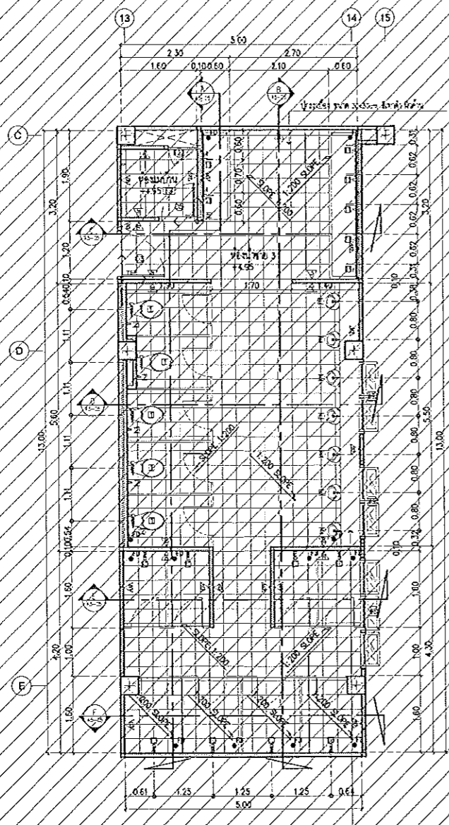
A5-05 แบบขยายห้องนอน 3 Scale 1:50
