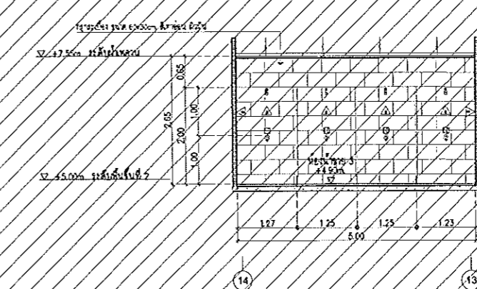
F แบบขยายรูปตัด Scale 1:50
