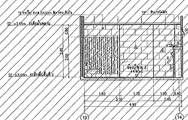
D แบบขยายรูปตัด Scale 1:50
