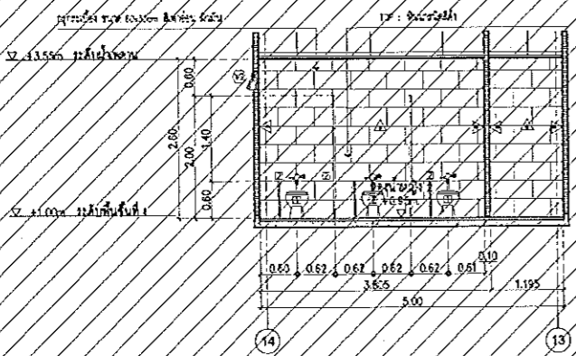
AS-04 AS-04 Scale 1:50 แบบขยายรูปตัด
