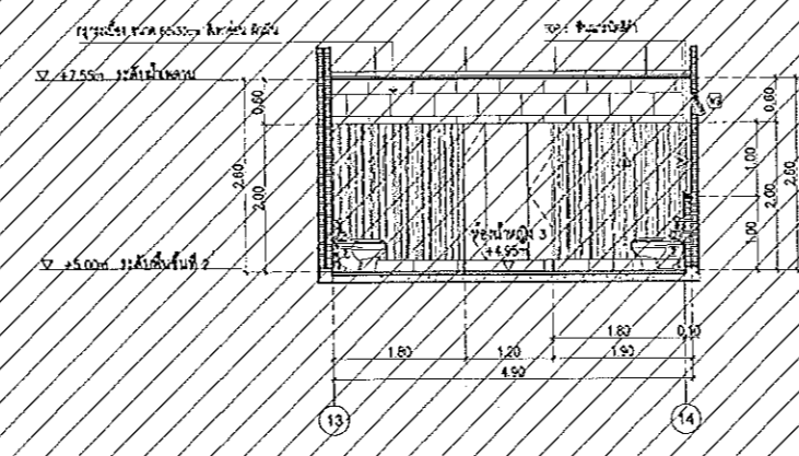
A5-06 แบบขยายรูปตัด Scale 1:50
