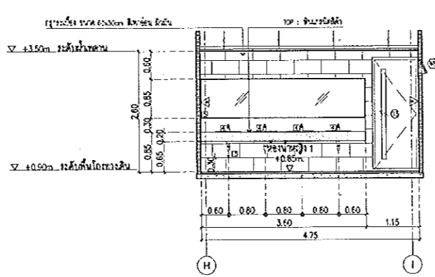
D แบบขยายรูปตัด A5-02 Scale 1 : 50
