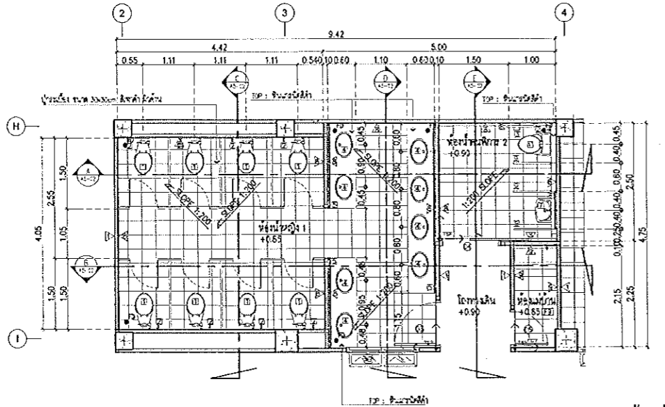
A5-02 แบบขยายห้องน้ำหญิง 1 Scale 1 : 50
