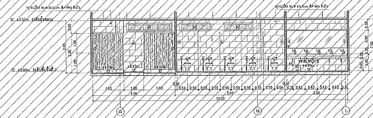
A5-06 แบบขยายรูปตัด Scale 1:50
