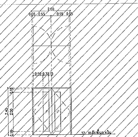
ELEVATION 02
