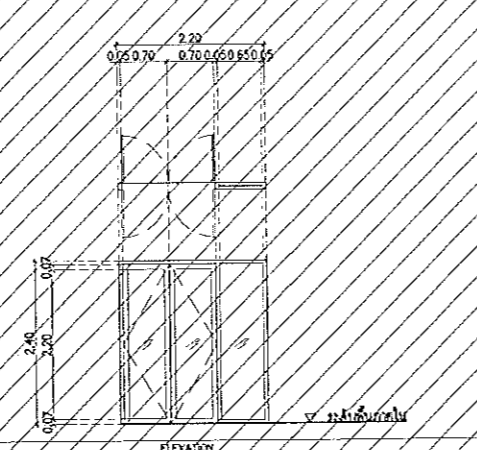
ELEVATION 06
