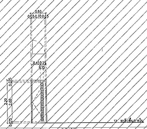
ELEVATION 05
