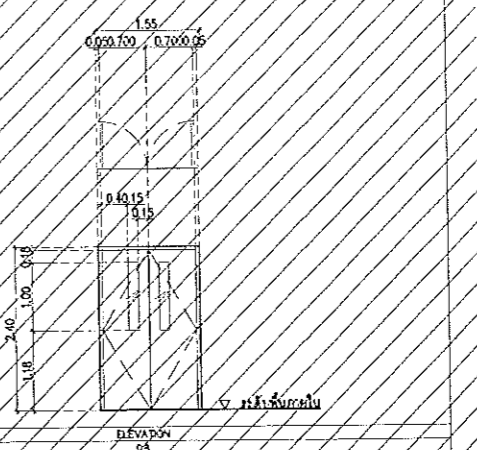
ELEVATION 08
