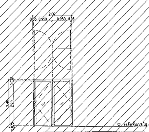
ELEVATION 09
