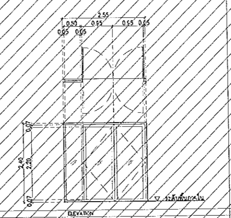
ELEVATION 07
