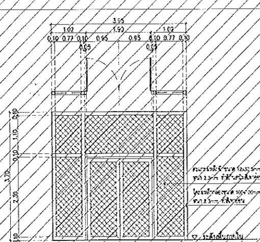
ELEVATION 01
