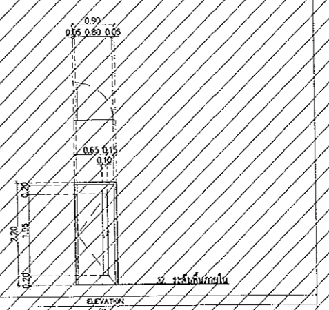
ELEVATION 12
