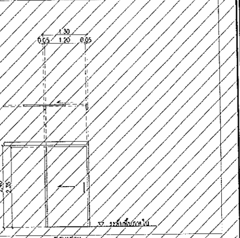
ELEVATION 04
